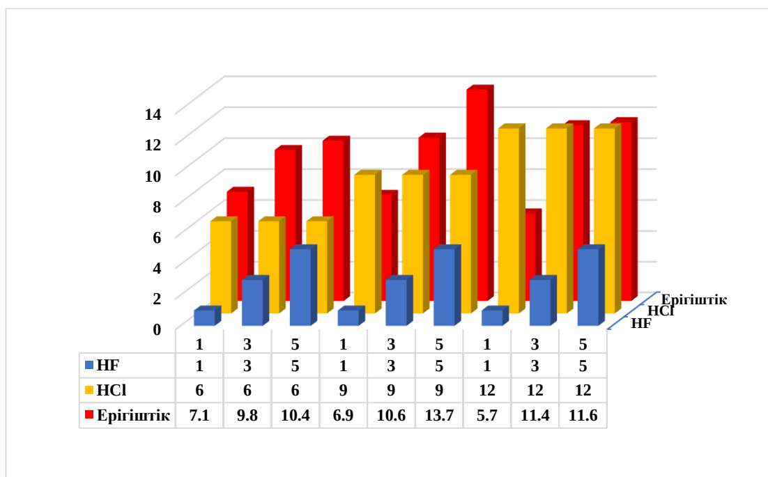
Сурет 4.4 – Тұз және гидрофтор қышқылдарының концентрациясына байланысты тау жыныстарының ерігіштігі мәндерінің орналасуы. Тау жынысы алынған тереңдік 324,50 м
