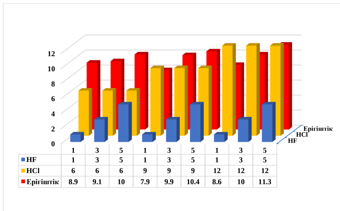
Сурет 4.9 – Тұз және гидрофтор қышқылдарының концентрациясына байланысты тау жыныстарының ерігіштігі мәндерінің орналасуы. Тау жынысы алынған тереңдік 352,21 м
