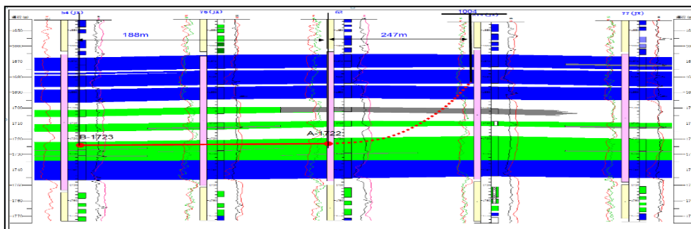
Рисунок Ошибка! Текст указанного стиля в документе отсутствует..1- Схема траектории горизонтального участка скважины 1004
