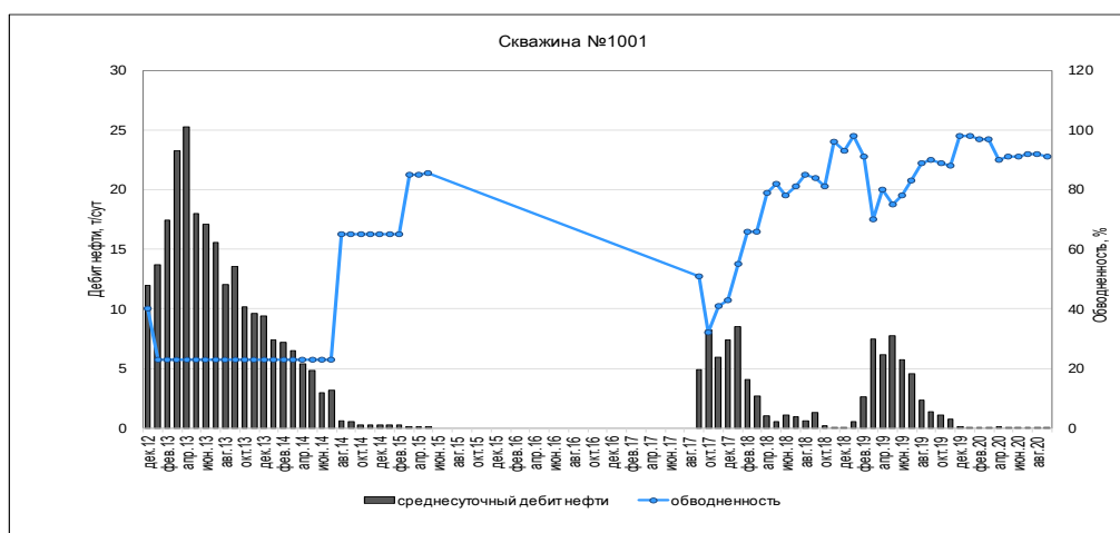
Рисунок Ошибка! Текст указанного стиля в документе отсутствует..8- График разработки горизонтальной скважины 1001
