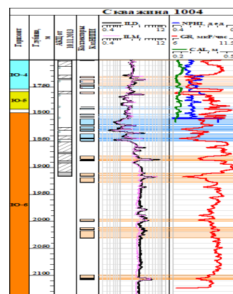
Рисунок Ошибка! Текст указанного стиля в документе отсутствует..2- Разрез скважины 1004 и изображение горизонтальной проекции скважины
