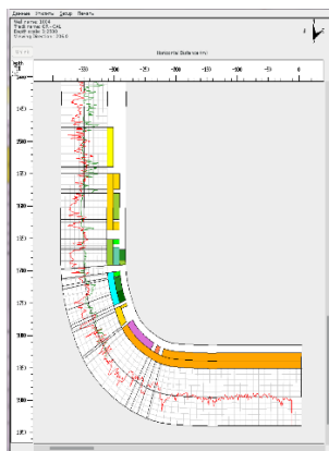
Рисунок Ошибка! Текст указанного стиля в документе отсутствует..2- Разрез скважины 1004 и изображение горизонтальной проекции скважины
