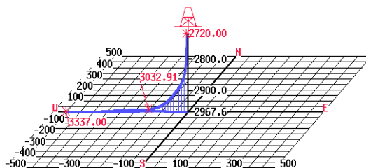
Рисунок Ошибка! Текст указанного стиля в документе отсутствует. -18 - Результаты 3Динклинометрии по скважине 25
