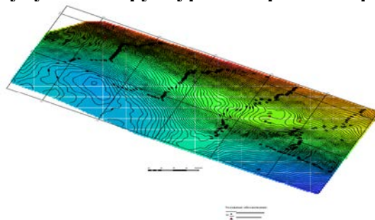
Рисунок 5. Улькендале Тучускен. Структурная карта по отражающему горизонту J_2k
