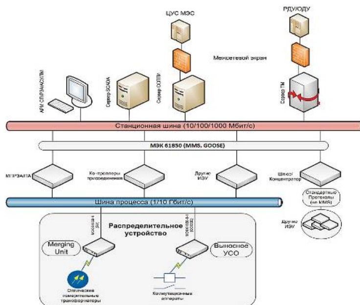
Рисунок 1 - Структурная схема цифрового программно-аппаратного комплекса подстанции
