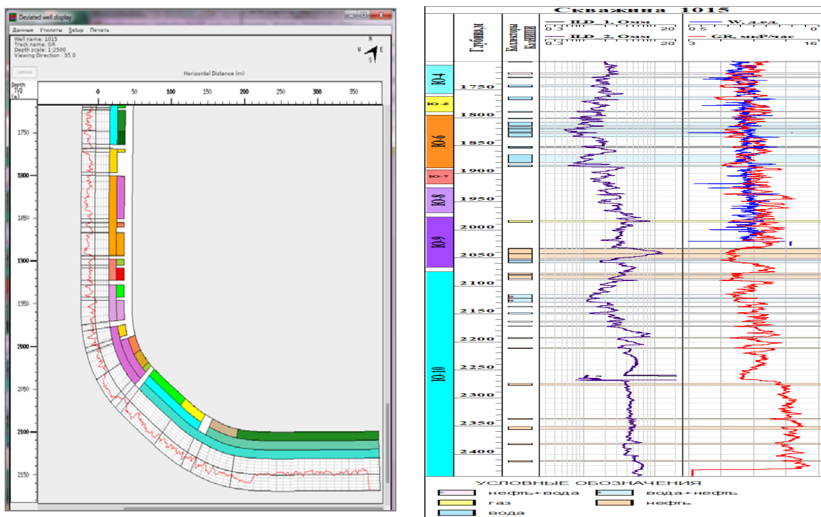
Рисунок Ошибка! Текст указанного стиля в документе отсутствует..6- Геофизическая характеристика пластов-коллекторов и фактическая горизонтальная проекция скважины 1015
