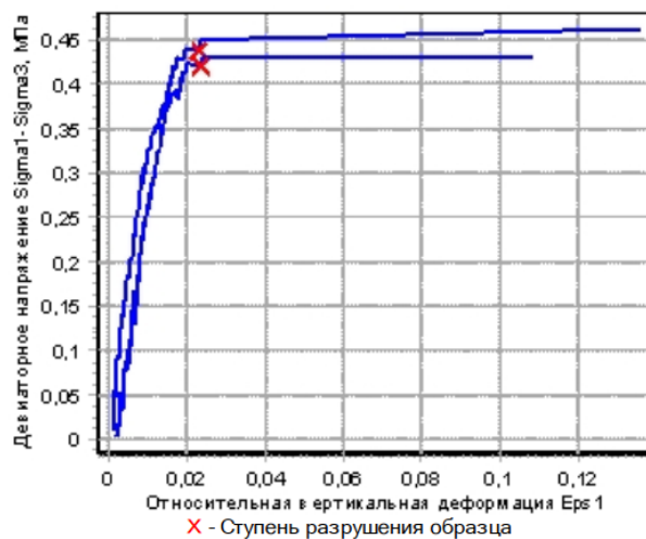
Рис. 3. График деформации образца в отношении к напряжениям
