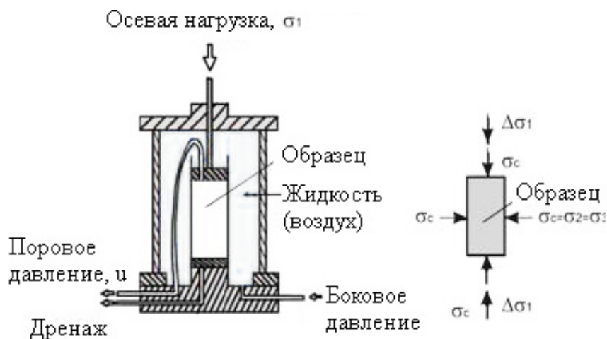
Рис. 1. Принципиальная схема Стабилометра типа Б
