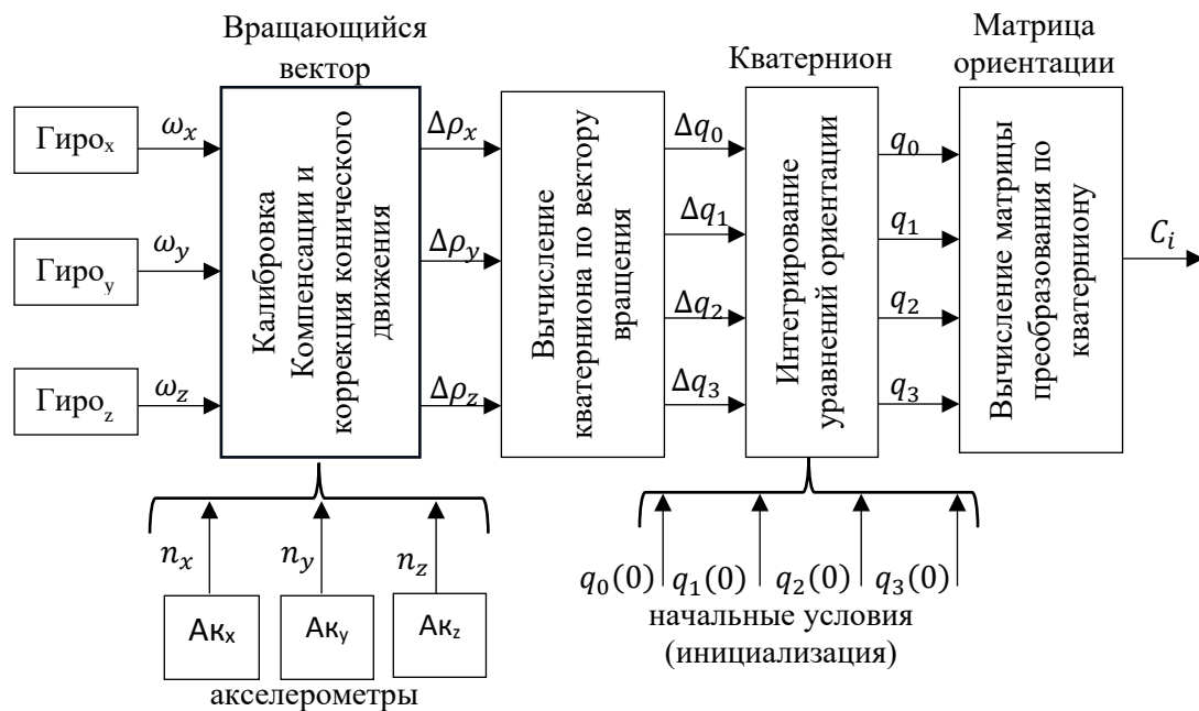
Рисунок 1 – Структурная схема преобразования данных вычисления ориентации
