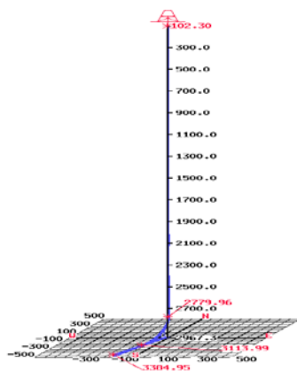
Рисунок 1 - Результаты 3D инклинометрии по скважине 26
