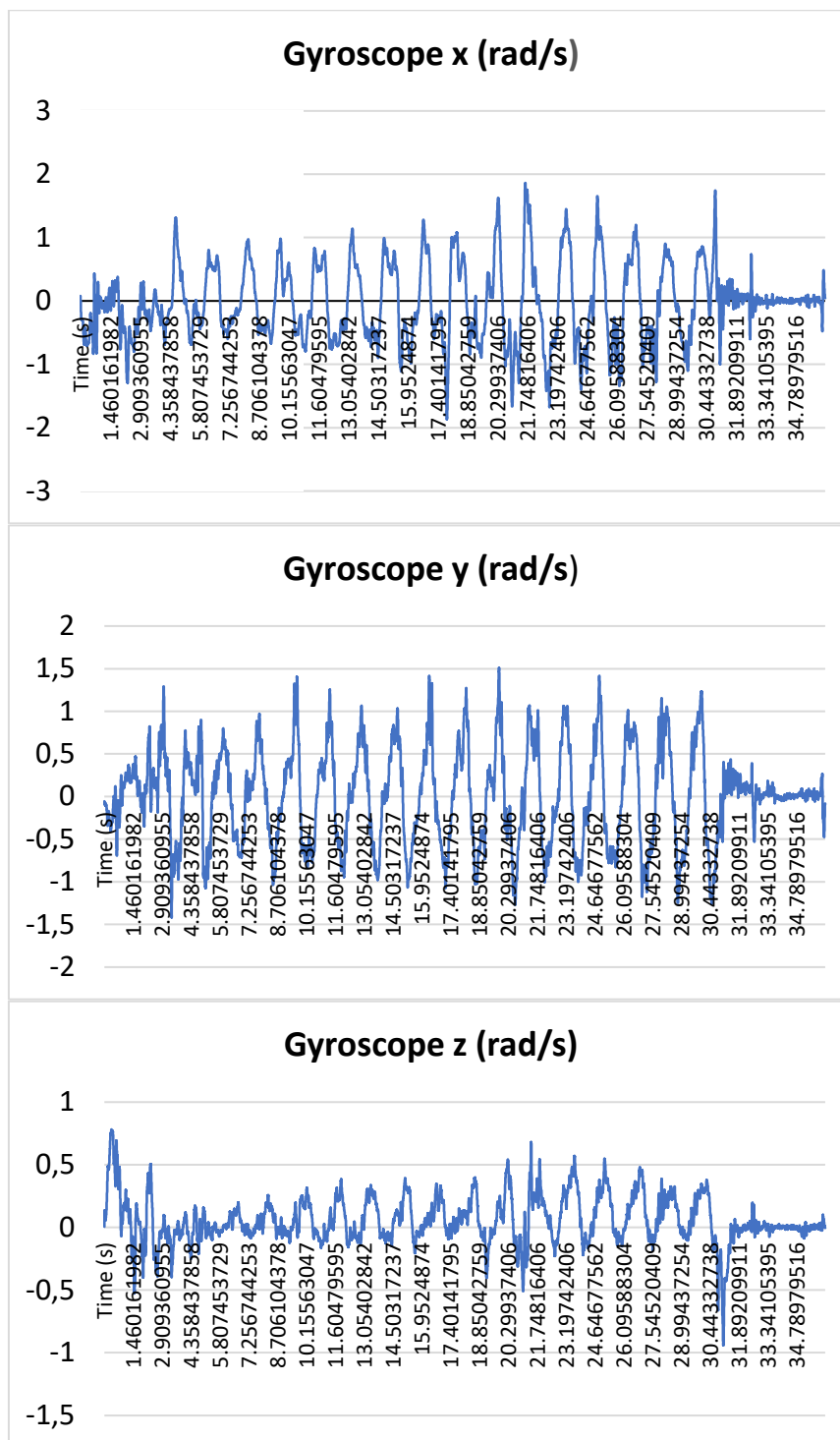
Рисунок 2 – Значения вычисленной динамики БЭС по осям x, y, z
