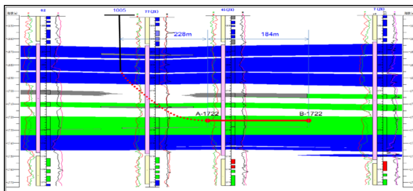
Рисунок Ошибка! Текст указанного стиля в документе отсутствует..5- Схема траектории горизонтального участка скважины 1015
